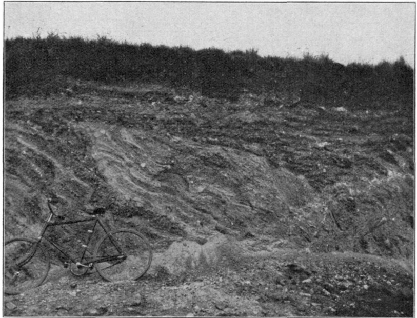
Abb. 6. / Aufschluß im Nordteil der Wiltschower Wallberge,
